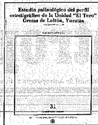
Estudio palinológico del perfil estratigráfico de la Unidad "El Toro" Grutas de Loltún, Yucatán. María Susana Xelhuantzi-López. Departamento de Prehistoria. Cuaderno de Trabajo núm. 31.
